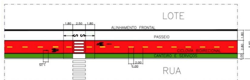
DETALHE CICLOVIA BIDIRECIONAL COM TRAVESSIA DE PEDESTRES S/ESC.
